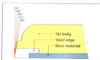
Side Edge Bevel
